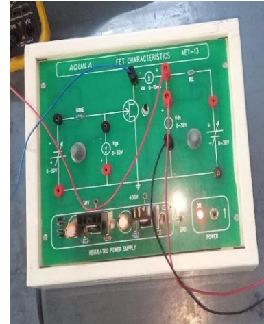
FET Characteristics
